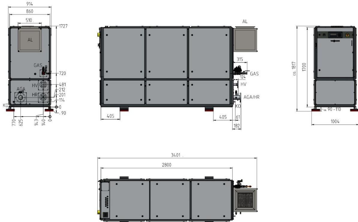
III. 5 Dimensions et raccords des modules de cogénération Vitobloc 200 EM-50/81 (dimensions en mm); Le boîtier de ventilateur déjà monté au dos peut être démonté pour l'installation du module
