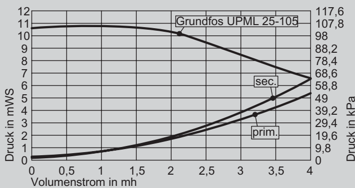
Pertes de charge de la station de déchargement Maxi DN 25
