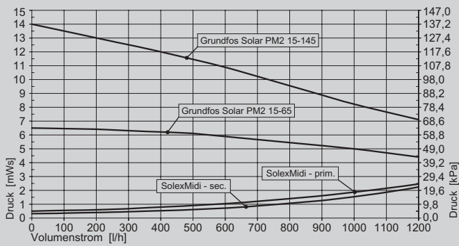
Pertes de charge de la station de transmission solaire Maxi DN 25
