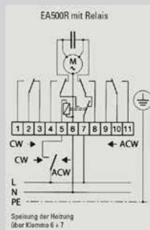
Schéma électrique EA500R
