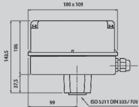
Servo-moteur EA500R
