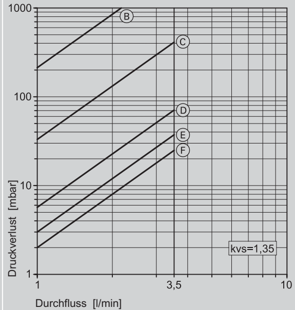
DN 15/1,0 - 3,5 l/mn
