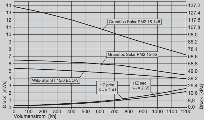
Pertes de charge de la station de transmission solaire Midi DN 20
