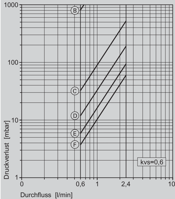
DN 15/0,6 - 2,4 l/mn
