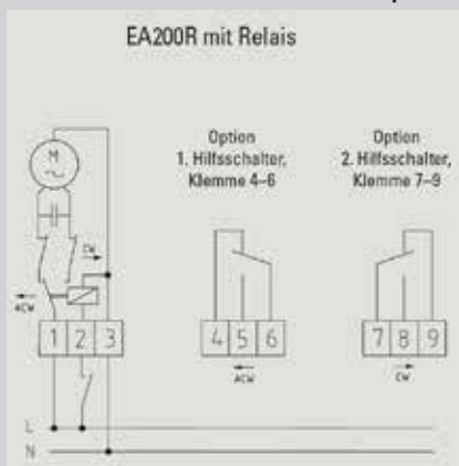
Schéma électrique EA200R
