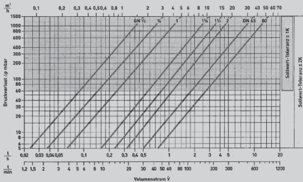
Diagramme des pertes de charge
