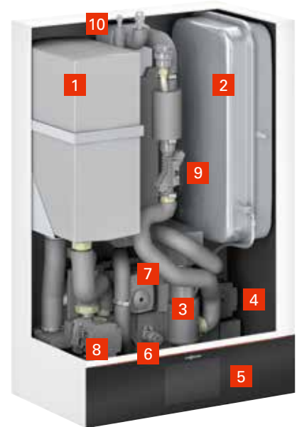
VITOCAL 200-S Mit zwei integrierten Heiz-/Kühlkreisen
